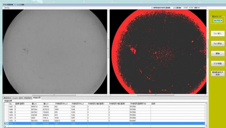
(上)SUTERUSU150V 装置外観 (左)高さムラを解析した画像。 赤色部分が高さムラの箇所
